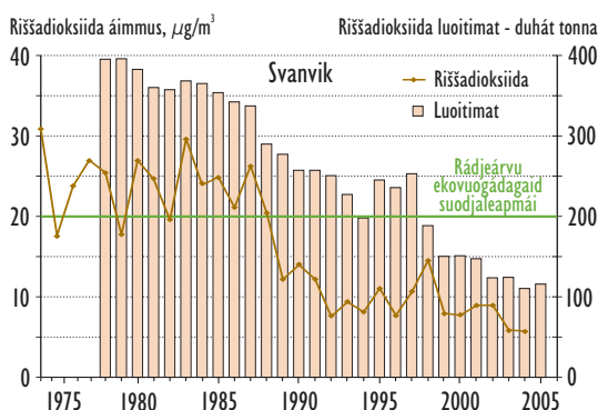
Gaskamearálaš jahkásaš riššadioksiidačoahkádus Svanvika áimmus orru unnume seamma leahtuin go šolgadanrusttegis unnot riššadioksiidaluoitimat.
