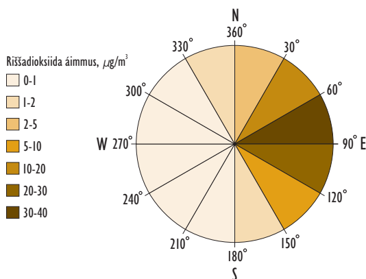
Svanvikas leat alimus riššadioksiidačoahkádusat dalle go lea nuortabiegga. Nuorta-davveoarji bieggas 2005/06 dálvvi dagahii ahte dálvvi gaskamearálašárvvu lei 13 alladeappot go dábálaš jagiin. Dakkár garra nuoskkiduvvon áimmu pulser bistet dábálaččat dušše moadde diimmu.
