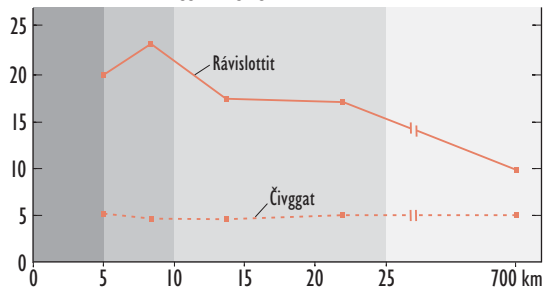
Veaikhehivodat báđođolggiin, mg/kg
