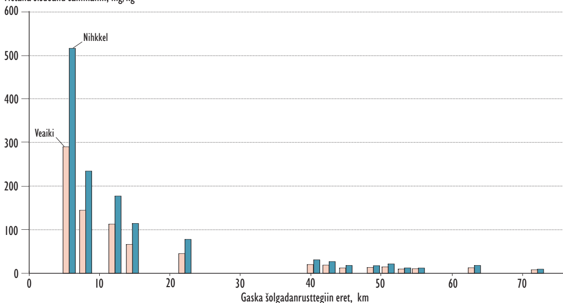
Metálla sisdoallu sámmáliin, mg/kg
