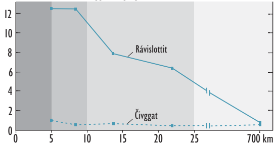
Nihkelhivodat báđođolggiin, mg/kg
