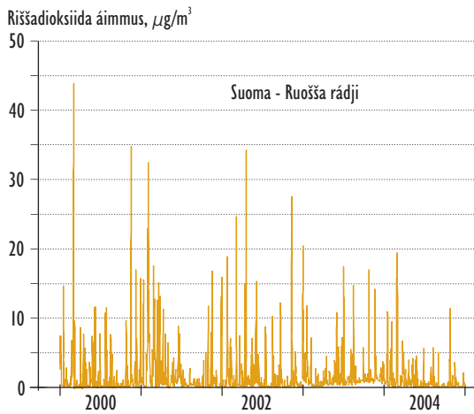
Raja-Jooseppi áibmomihdanstašuvdna Suoma-Ruošša rájjs registrerii 15 luoitima 2002:s. Nu ollu nuoskkidančoahkádusat leat hárvve industriáliserejuvnon guovlluin ja eai oidno bájjo goassege Suoma eará referánsaguovlluin.
