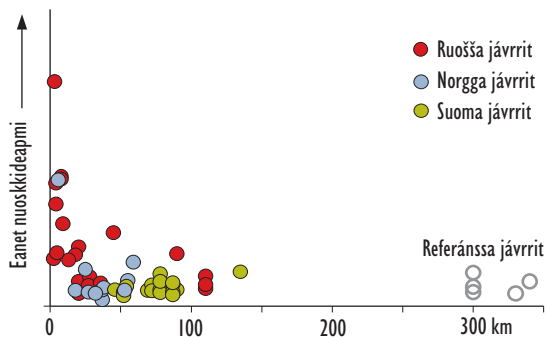
Lossametállat leat garrasit nuoskkidan jávresedimeantaid lagamus 10 kilomehtara šolgadanrusttegis eret. Dábálaš árvvuid gávdná easka sullii 50 km rusttegis eret.
