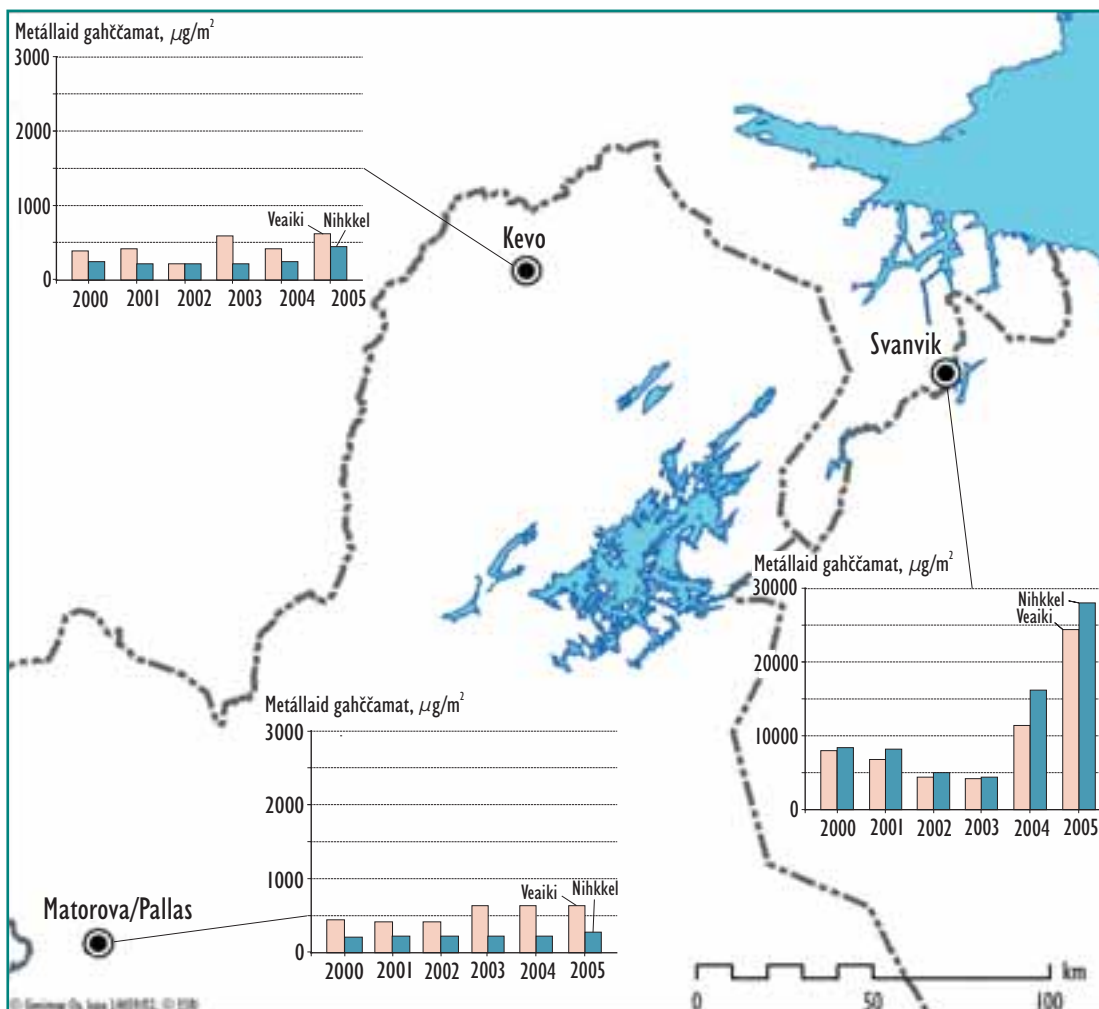
Čájehuvo ahte veaikki ja nihkkela gahččamat leat jagi 2000 rájes lassánan sihke hui lahka šolgadanrusttegiid ja referánsastašuvnain nu guhkkinis eret go Kevos.
