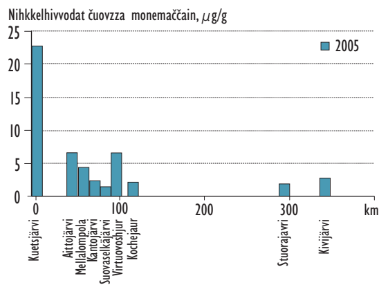
Nihkkelčoahkádus čuo- vžžaid monemaččain unnu jođánit mađi guhkkelis eret rusttegis lea, muhto orru duppalastojuvvon golmmajagáš áigodagas guovllus mii lea 100 km Nikela lulábealde.
