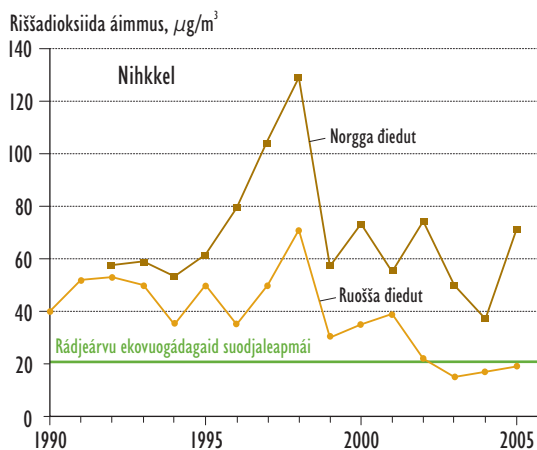
Ruošša gozihandieđut čájehit ahte Nikela riššadioksiidačoahkádusat leat 2002 rájes leamašan ekovuogádagaid bisuheami rádjeárvvu dásis dahje vuollel dan. Norgga gozihandieđut čájehit baicca ges ahte Nikela riššadioksiidačoahkádusat leat badjel golmma geardde eanet go mearriduvvon rádjeárvvu. Lea dárbu lagabui čielggadit manin dát guokte diehtočoakkáldaga leat nu guovtteláganat.
